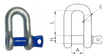
Скоба G210
